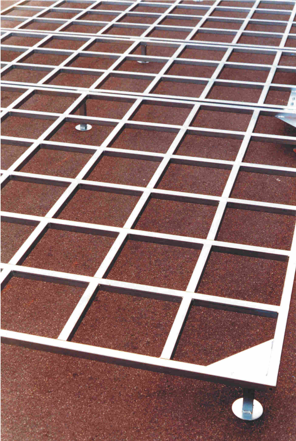
Plateforme galvanisée à chaud pour les aires d'atterrissage en saut en hauteur, hauteur du sol cm. 20
